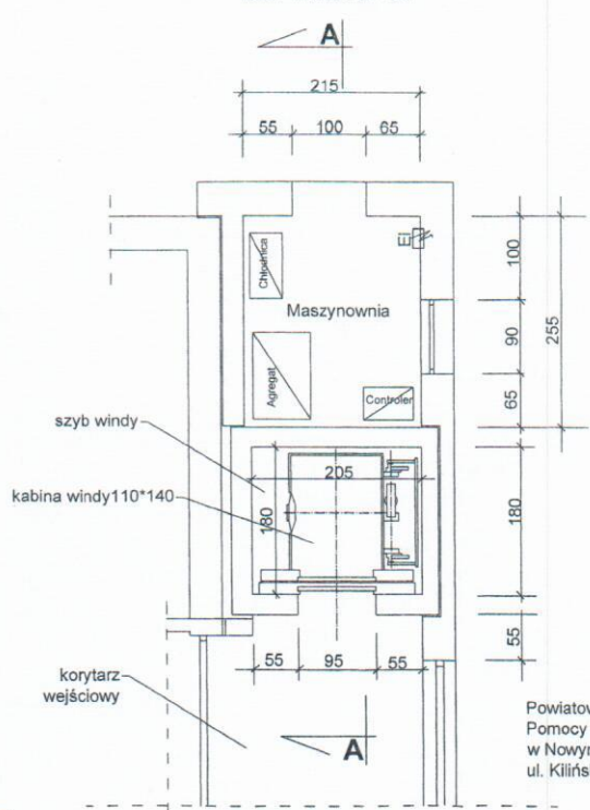
RZUT PARTERU 1:50
